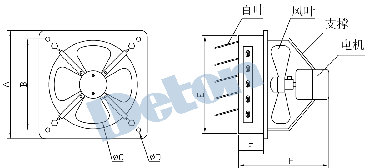
外形结构图
